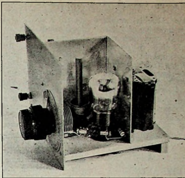
De generator-detector met de korte-golf-afstem-middelen. Zie voor Bouwschema R.E. No. 21 en 22.
