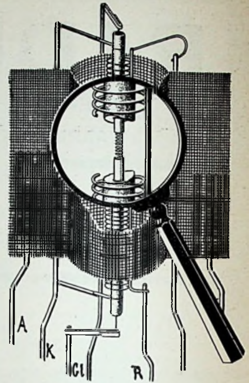
Doorsnede door het systeem eener indirect verhitte Telefunken-gelijkstroomlamp.
