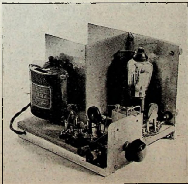
De aperiodische hoogfrequenttrap, middelfrequent-koppelkring en gloeistroomtransformator.
